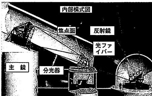
LAMOST外観と内部模式図 (下/提供：中国科学院国家天文台)
